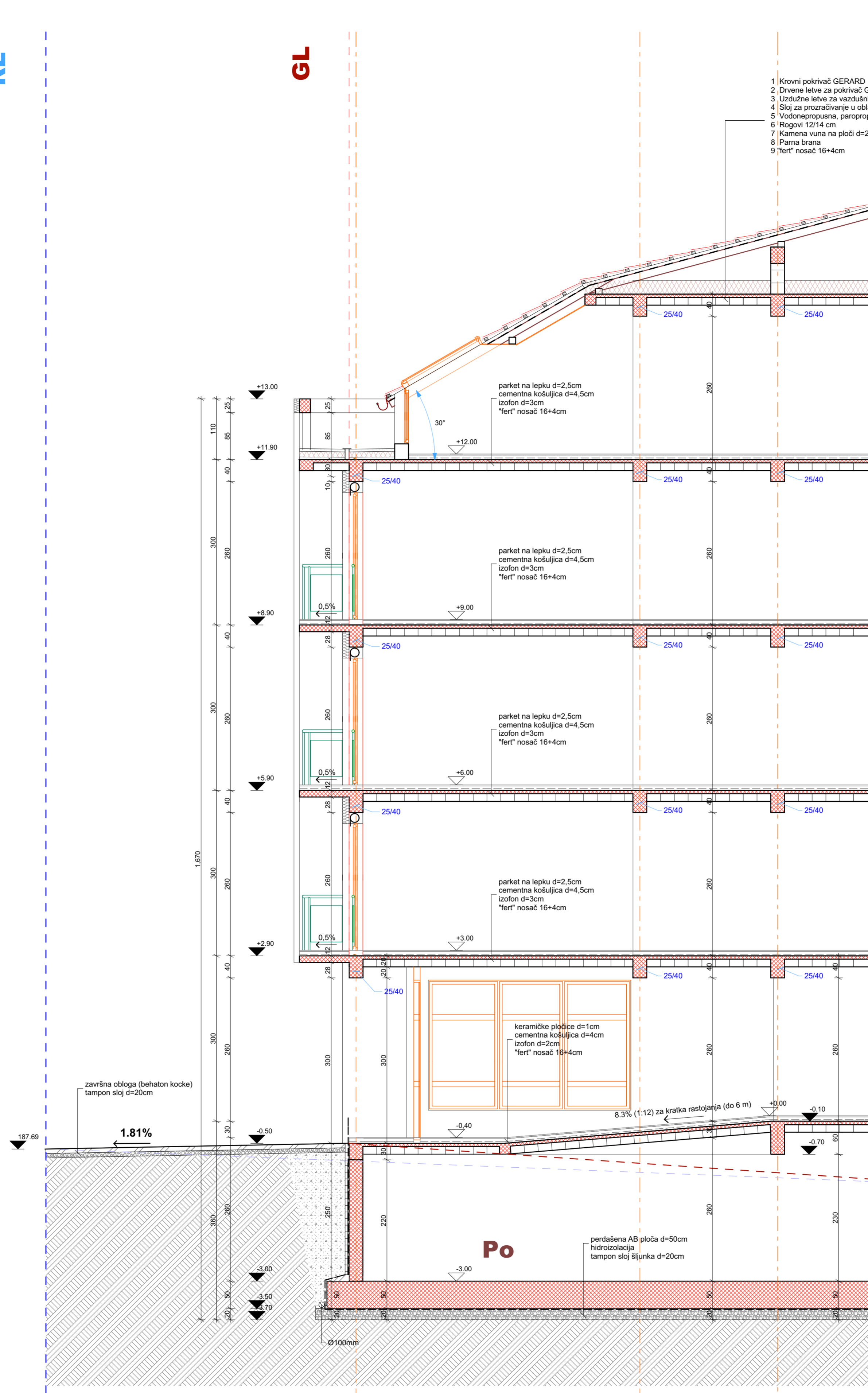
PRESEK 3-3
