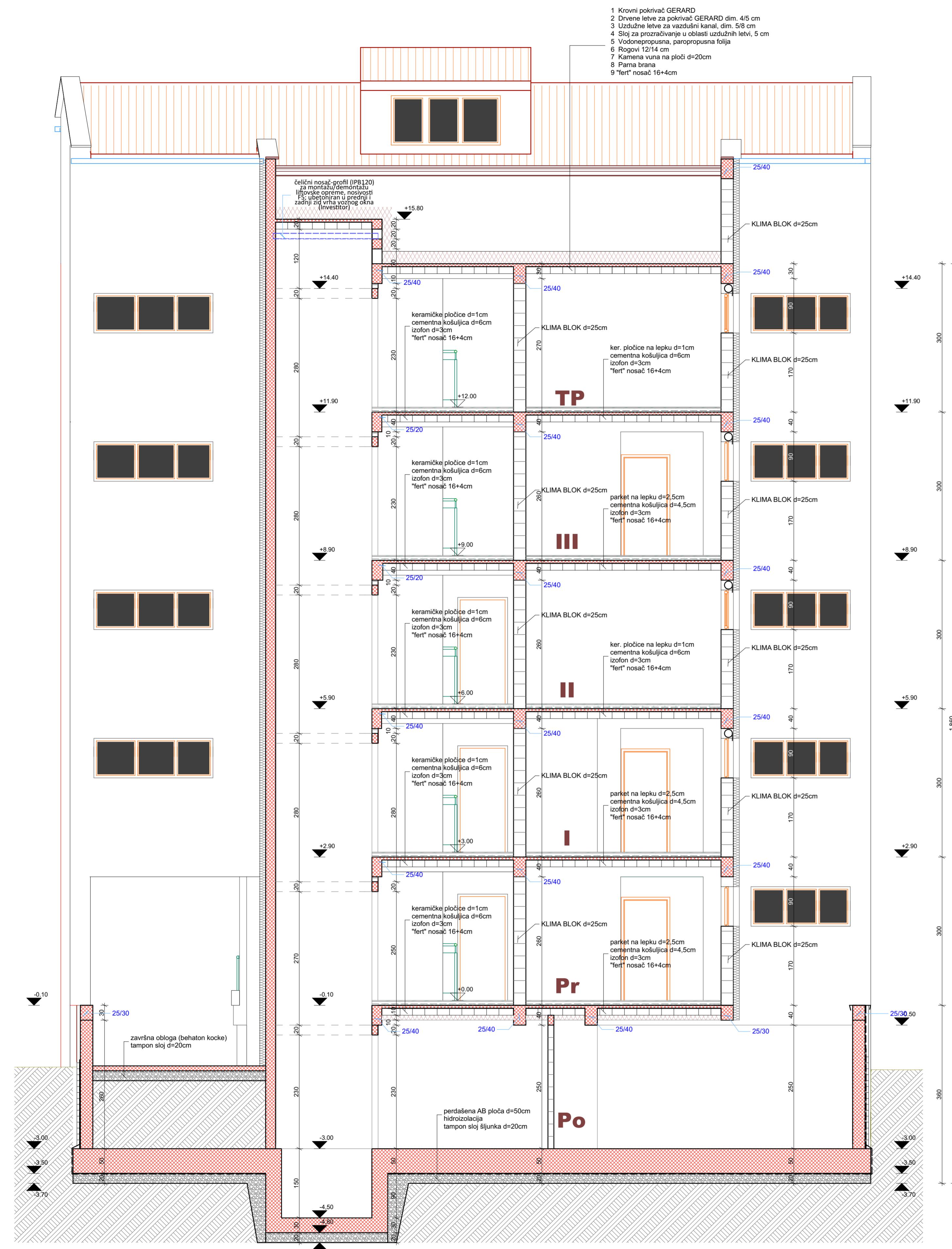
PRESEK 2-2
