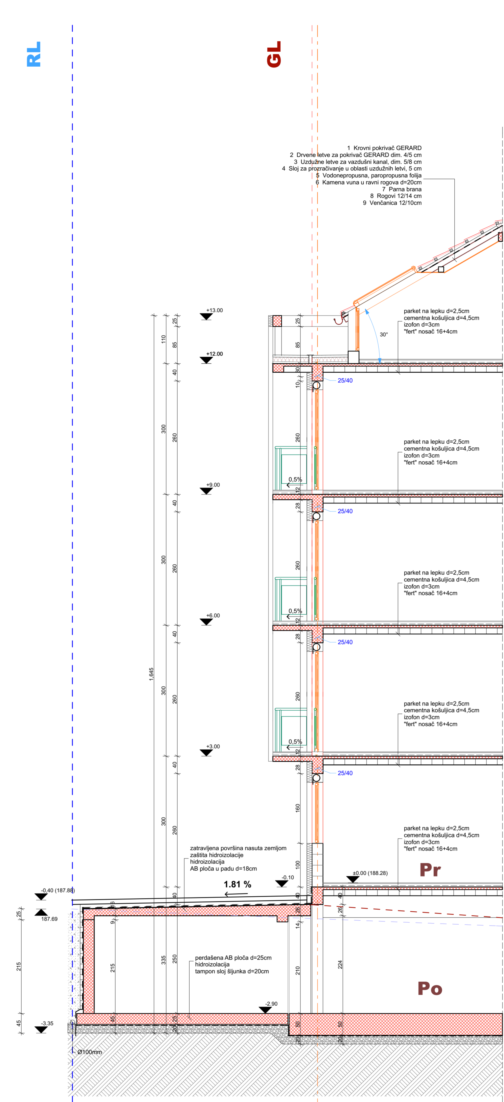
PRESEK 4-4
